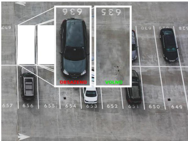
Klasifikace výřezu
